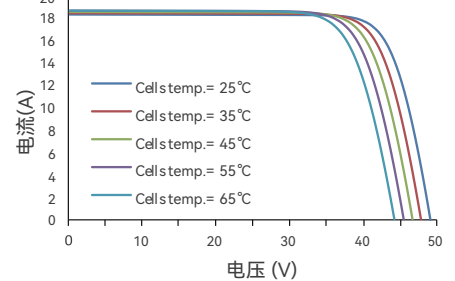
电流-电压曲线(725W)
